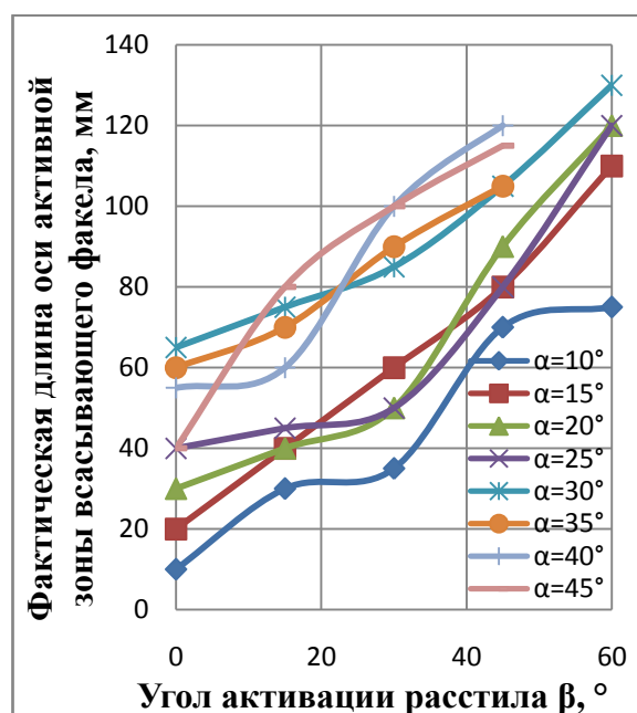
Рисунок 10 – Зависимость длины оси активной зоны всасывающего факела от угла установки сопла \alpha и переднего угла мундштука (угла активации расстила) \beta для верхового (а) и переходного (б) торфа
