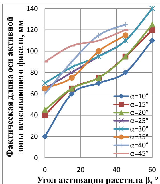
Рисунок 10 – Зависимость длины оси активной зоны всасывающего факела от угла установки сопла \alpha и переднего угла мундштука (угла активации расстила) \beta для верхового (а) и переходного (б) торфа
