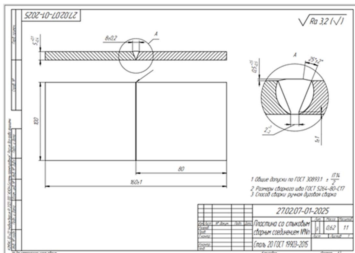
Рисунок 1 – Чертеж пластины
