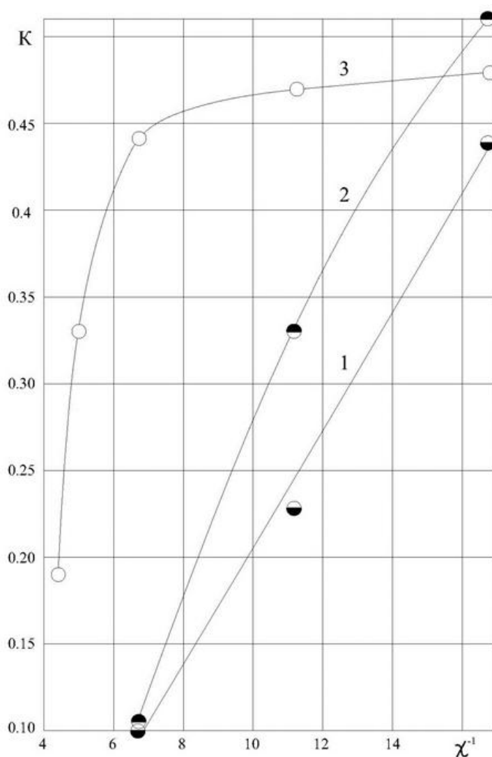
Рисунок 3.6. Зависимость однородности эмульсии от обратной величины критерия кавитации при \delta , мм: 1 – 0,07; 2 – 0,14; 3 – 0,21
